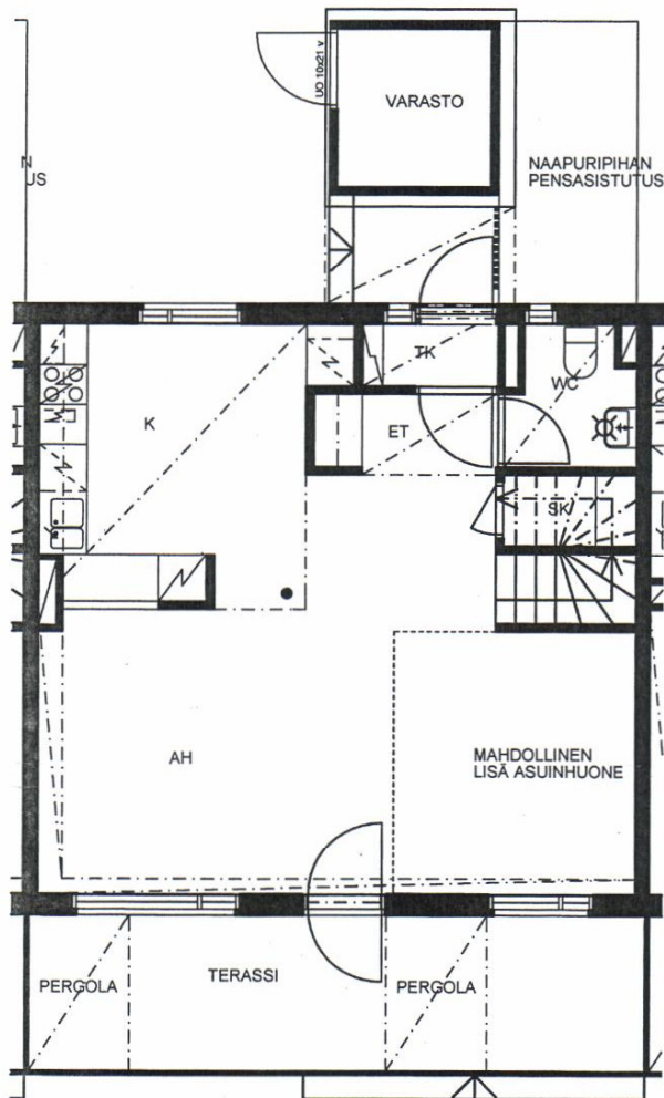
1.KERROS
