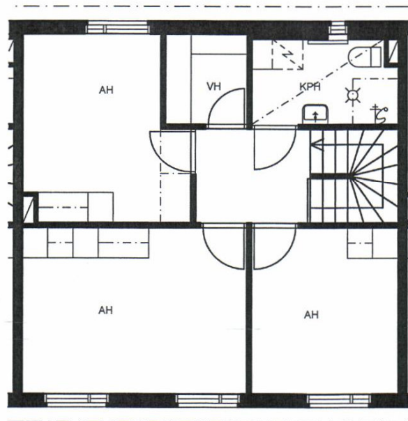
2.KERROS
