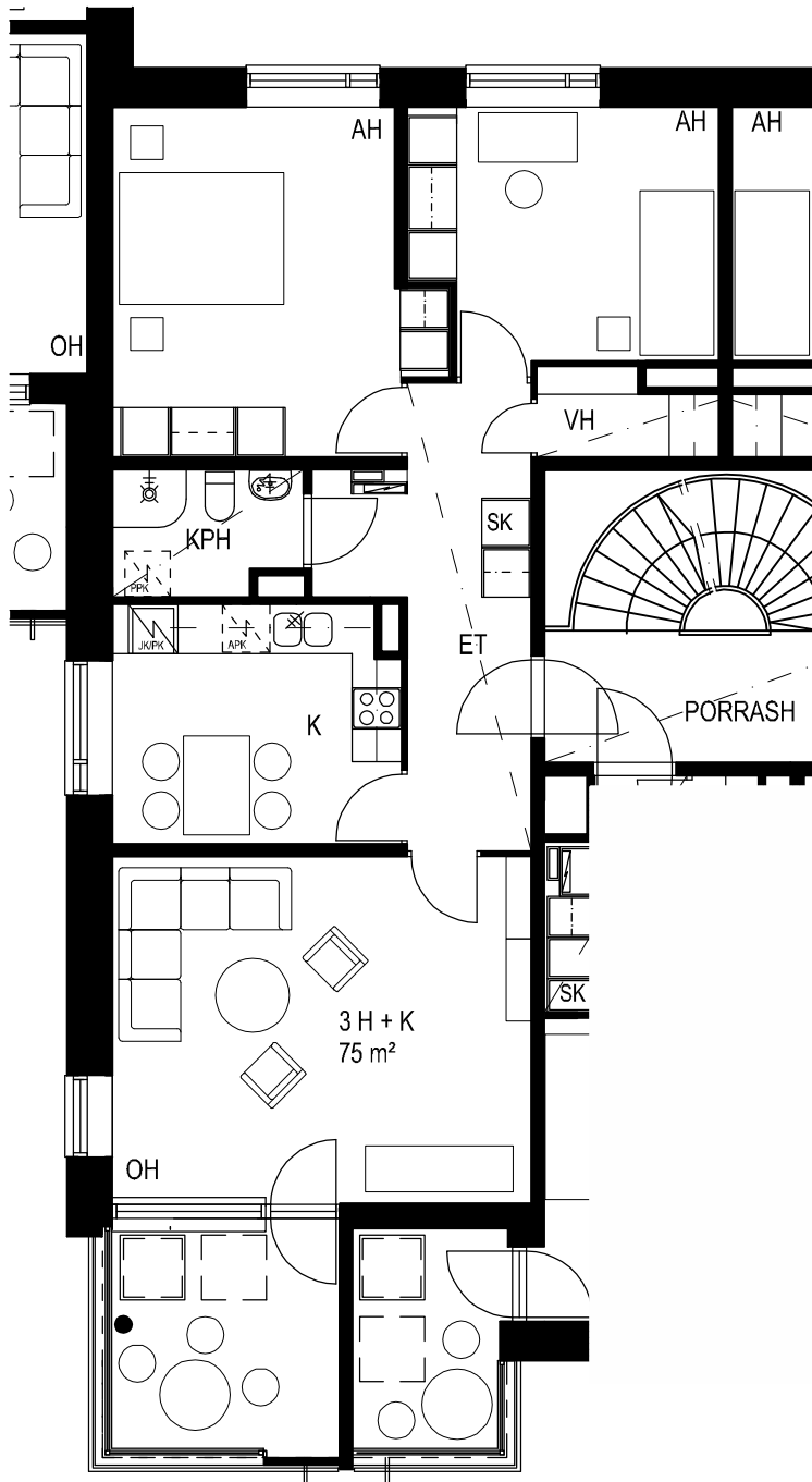
HUONEISTOPIIRROS 1:100
