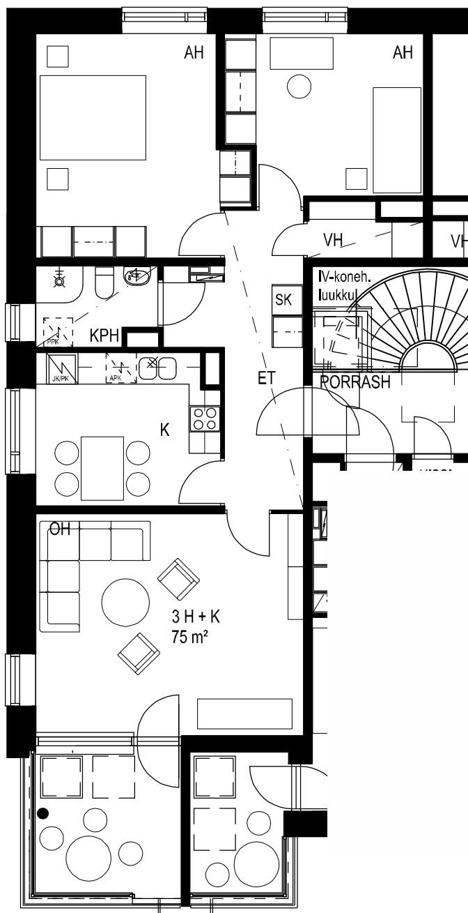
HUONEISTOPIIRROS 1:100
