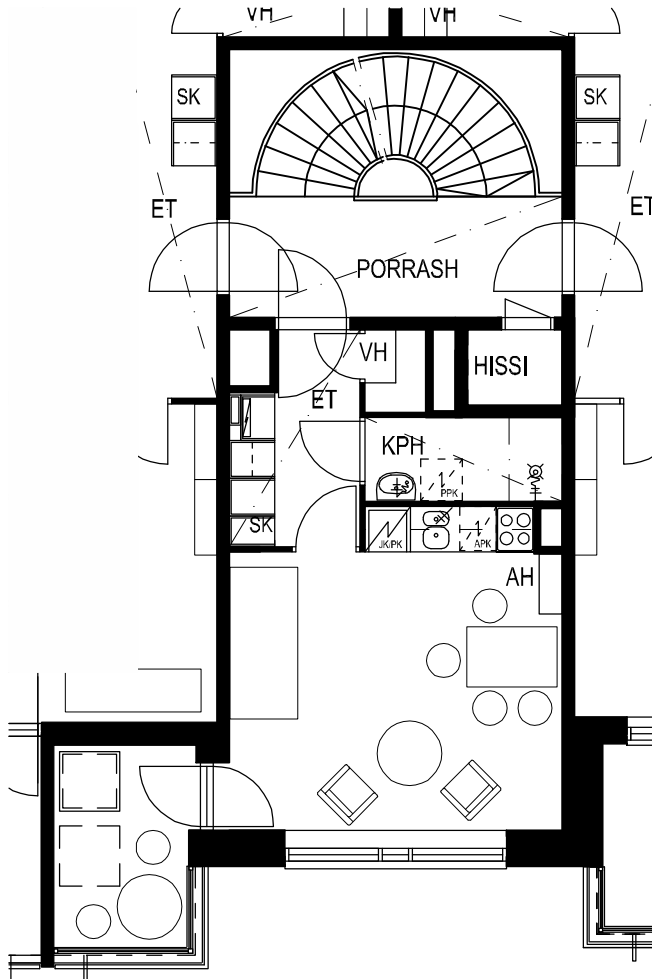
HUONEISTOPIIRROS 1:100
