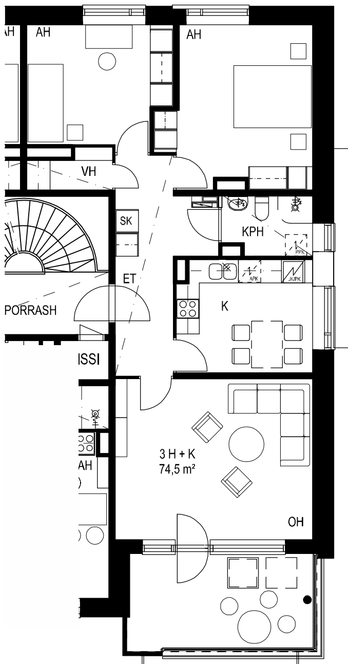
HUONEISTOPIIRROS 1:100
