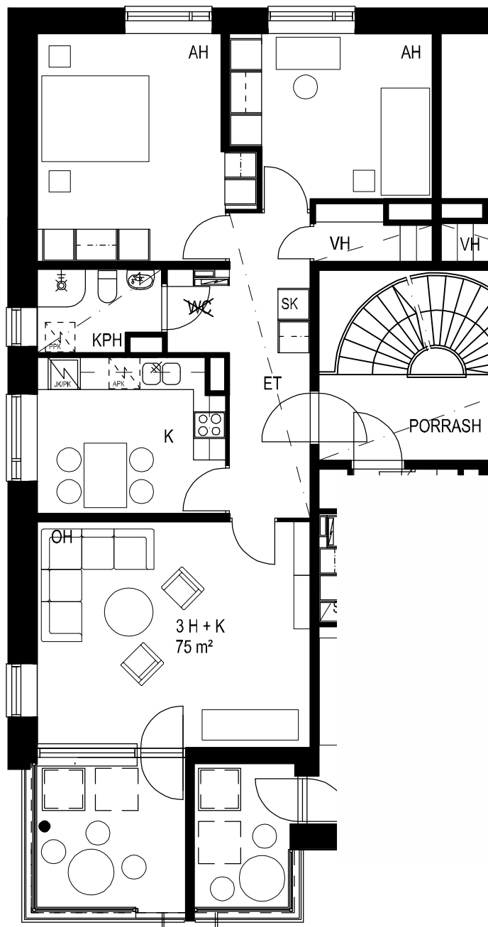
HUONEISTOPIIRROS 1:100
