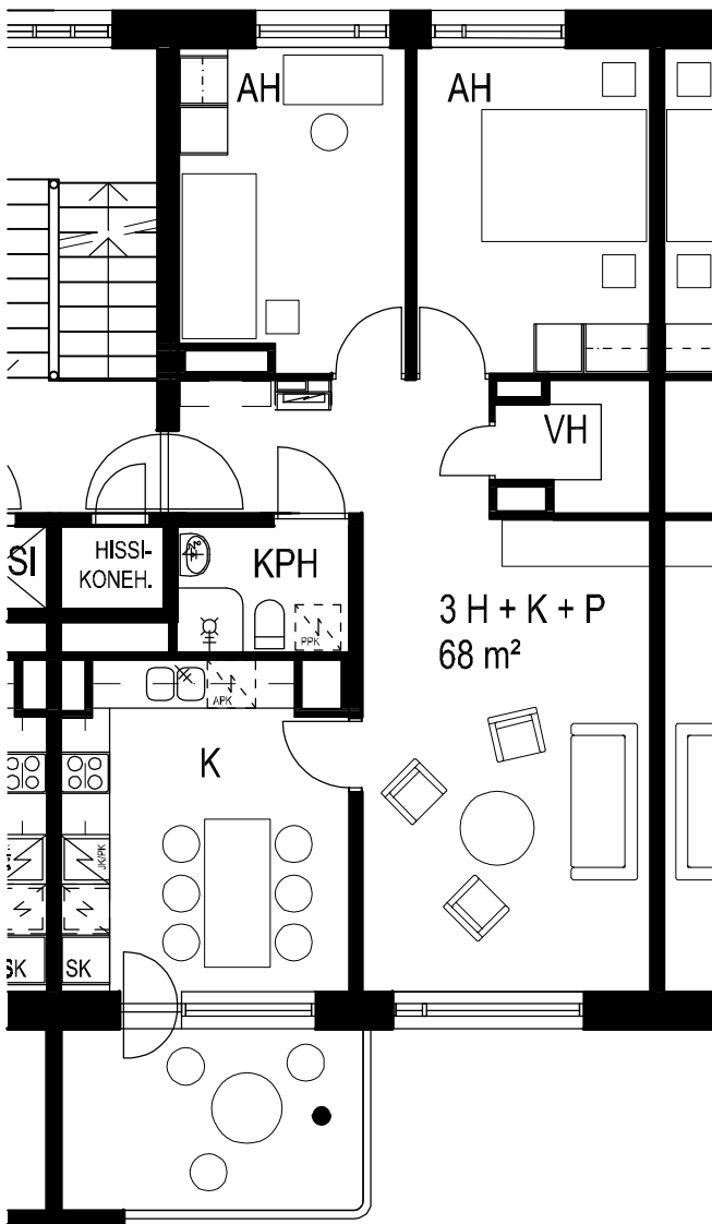
HUONEISTOPIIRROS 1:100
