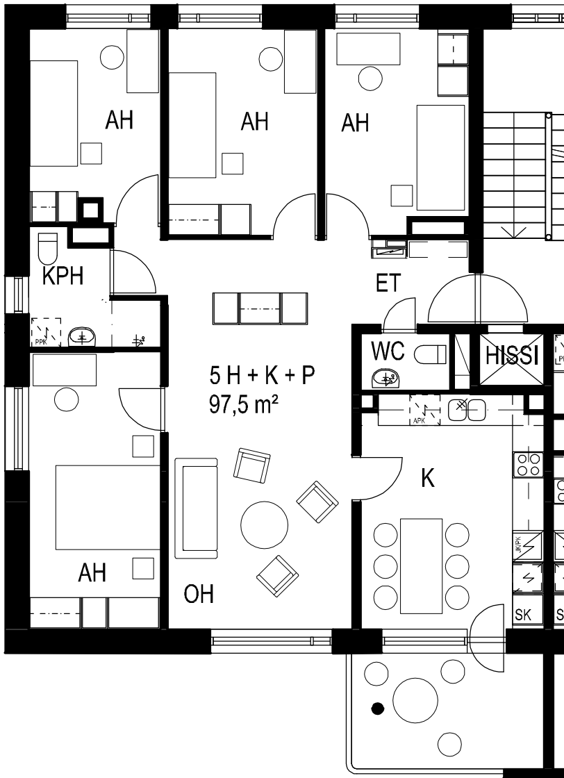
HUONEISTOPIIRROS 1:100
