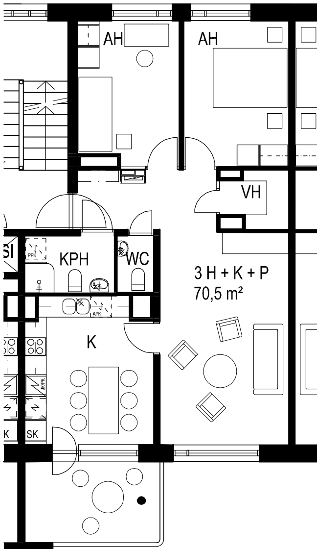
HUONEISTOPIIRROS 1:100
