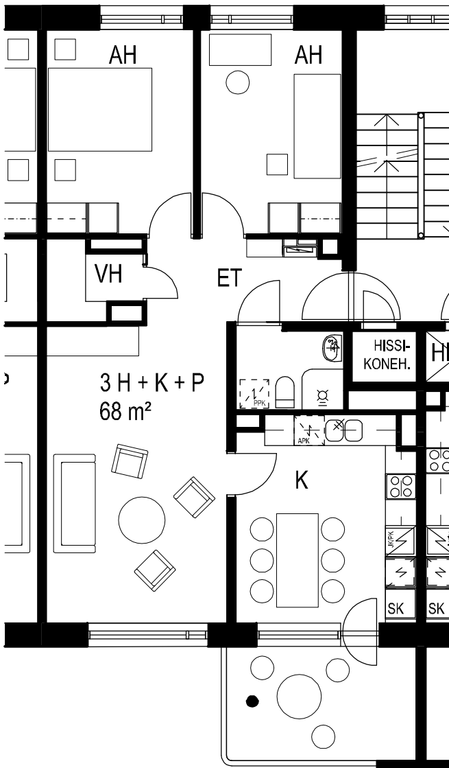
HUONEISTOPIIRROS 1:100
