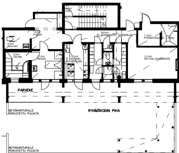
1. KERROS POHJA 1/250
