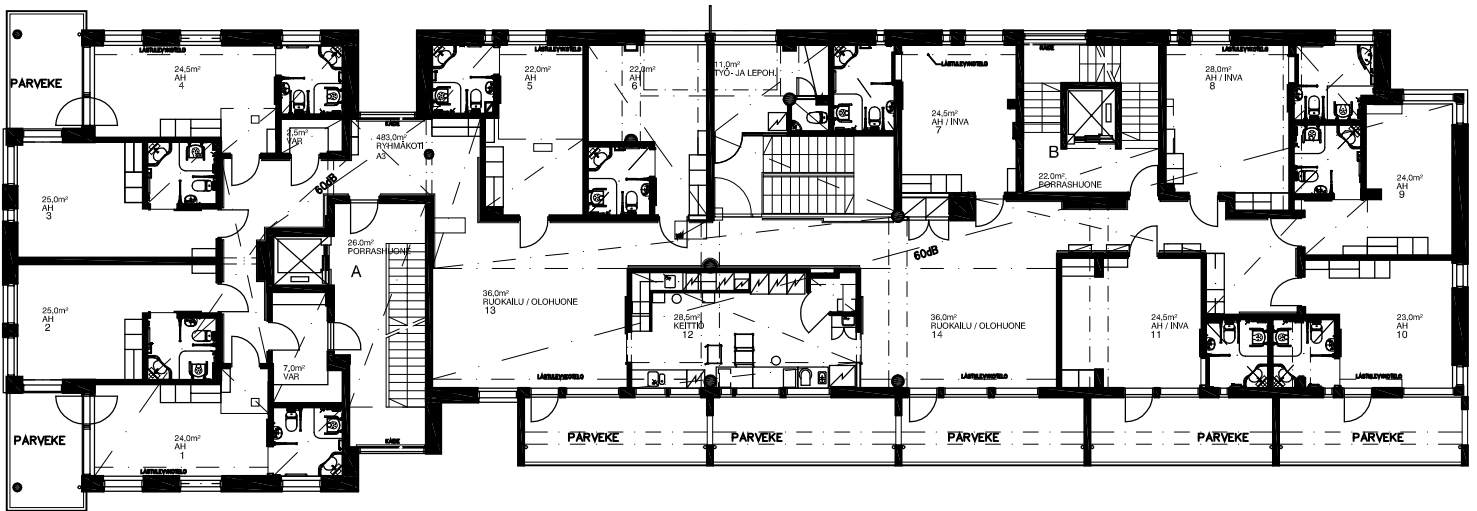
2. KERROS POHJA 1/250
